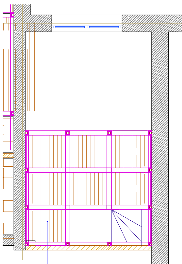
План полов 2 уровень
