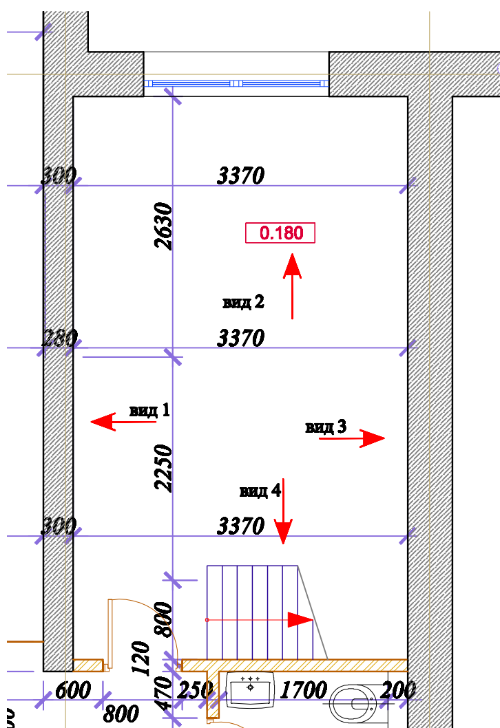
План разверток
