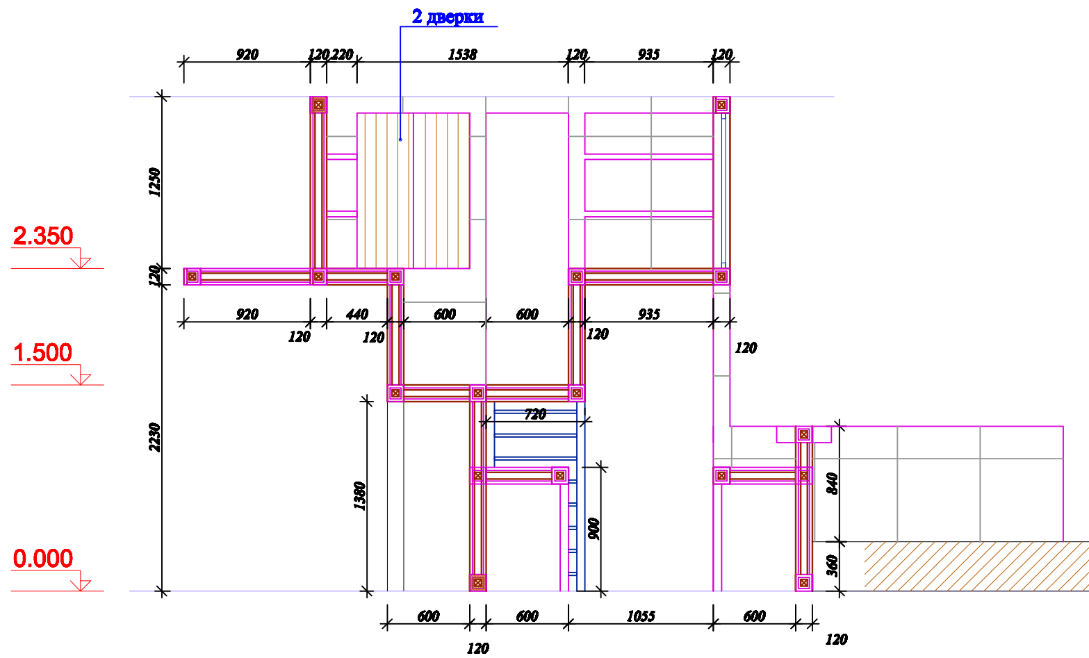
Разрез 2-2
