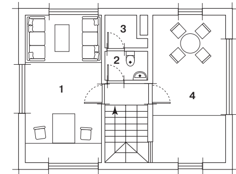
План мансардного этажа
